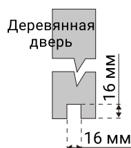
Размер фрезеровки для профиля AIR SOFT 03
